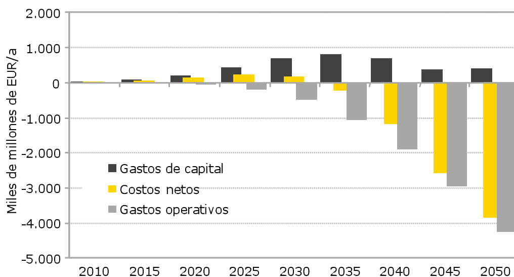
Gráfica 6 - 14 Resultados para el transporte - infraestructura.
