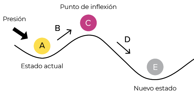
Figura 2.1 Un sistema se mantiene en su estado actual (A, círculo amarillo) aunque se produzcan continuamente cambios a pequeña escala, siempre que pueda absorber las presiones (o motores del cambio). Sin embargo, la presión (B) puede llevar a un sistema a su límite o punto de inflexión (C, círculo rosa) de forma gradual o mediante un choque. Cuando un sistema alcanza un punto de inflexión, el cambio se acelera (D) hasta alcanzar un nuevo estado (E, círculo gris) 55 .
